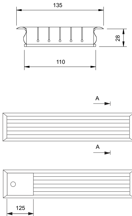
Leikkaus A-A
