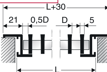
PITKITTÄISLEIKKAUS
