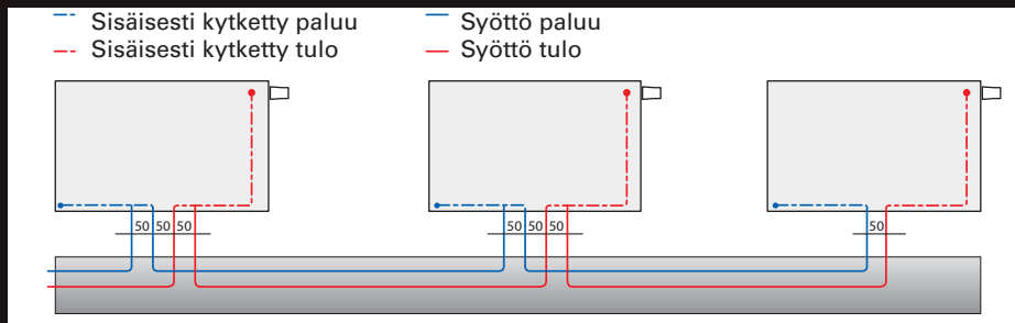
Periaatekuva MODUL4:n asentamisesta.
